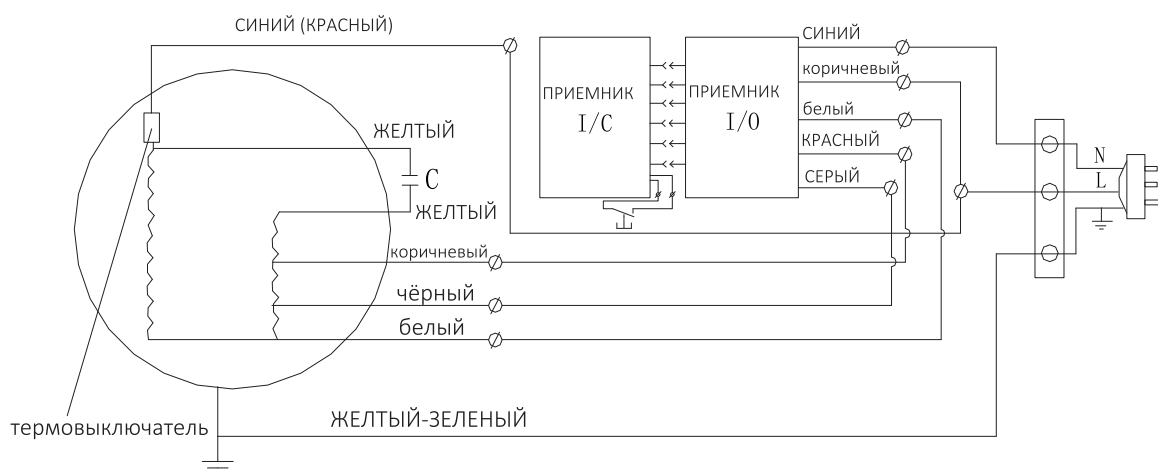
ТРЕХСКОРОСТНОЙ ПЕРЕКЛЮЧАТЕЛЯ СХЕМА СОЕДИНЕНИЙ
